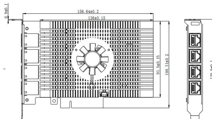
Dimensions (unit:mm)
